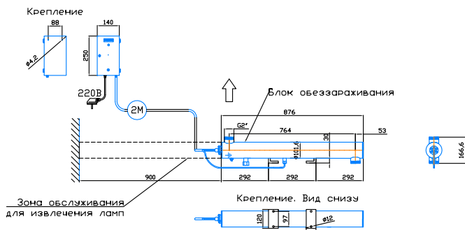
Монтажный чертёж установки ОДВ-10 (ОДВ-4С). Патрубки - И. Изготовление под заказ. Горизонтальное расположение
