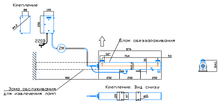
Монтажный чертёж установки ОДВ-10 (ОДВ-4С). Патрубки - П. Изготовление под заказ. Горизонтальное расположение
