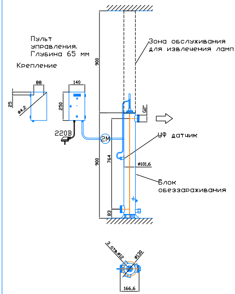
Монтажный чертёж установки ОДВ-10 (ОДВ-4С) Патрубки - И. Стандартное изготовление Вертикальное расположение
