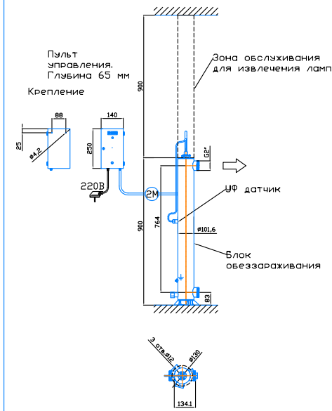
Монтажный чертёж установки ОДВ-10 (ОДВ-4С) Патрубки - П. Изготовление под заказ Вертикальное расположение
